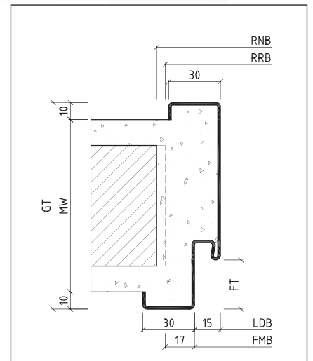
standard tok kőműves falhoz
