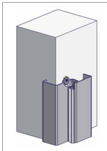
Saroktok átlós rögzítéssel
