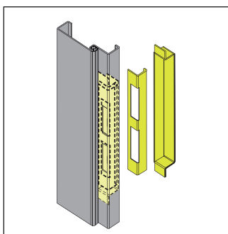
Erősített zárlemez: A betörésbiztonság és a tartósság növelésére.
