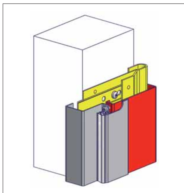
Typ K, 2részes, falvastagságában állítható -5 - +15 mm-t
