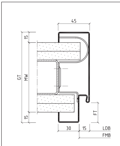
standard tok gipszkarton falhoz
