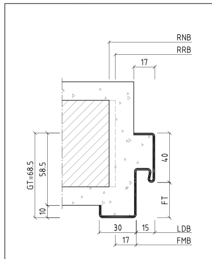
standard saroktok kőműves falhoz
